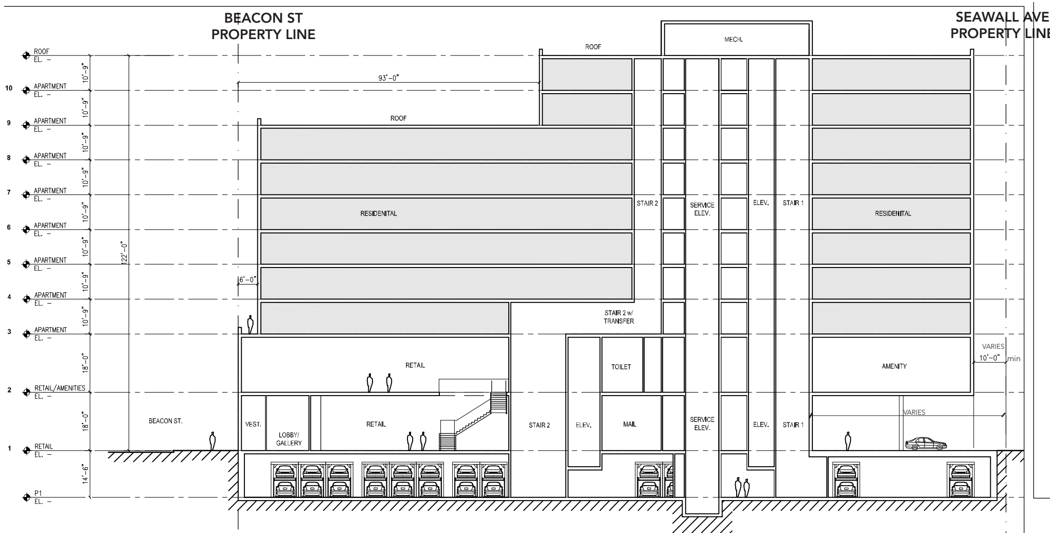
SECTION A-A
